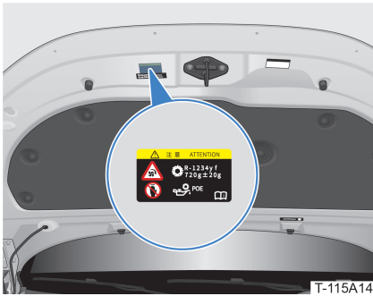
Warnaufkleber für Kältemittelauffüllung und Kühllüfter
