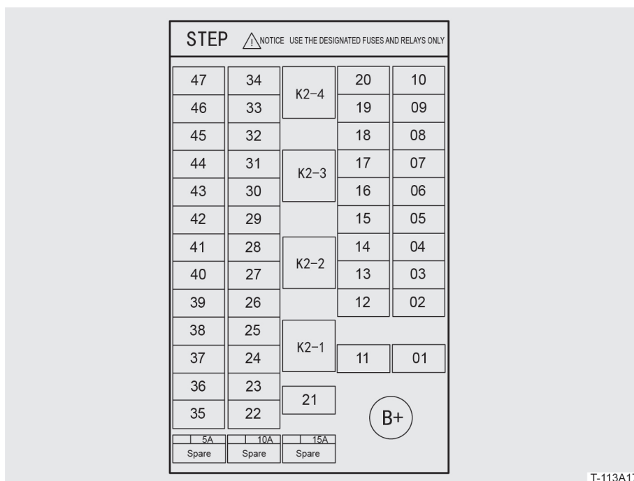
Verteilung der Armaturentafel-Sicherungskästen
